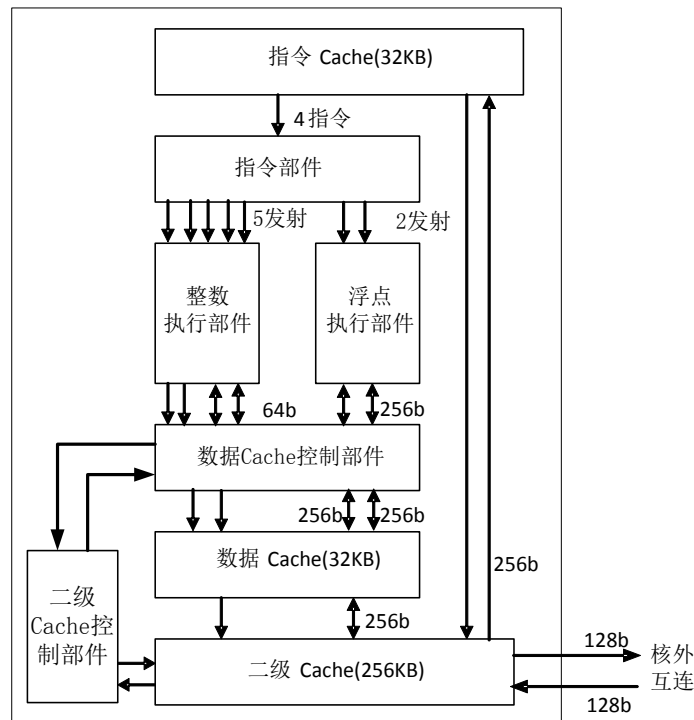
图 1-1 SW421 核心结构框图
