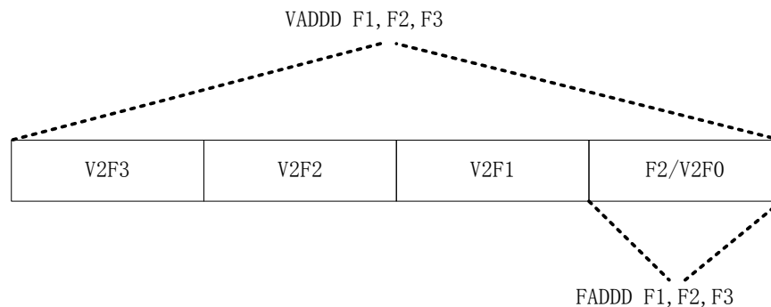
图 11-2 浮点寄存器和向量寄存器在使用中的差别
