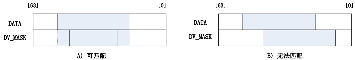
图 10-1 匹配情况示例
