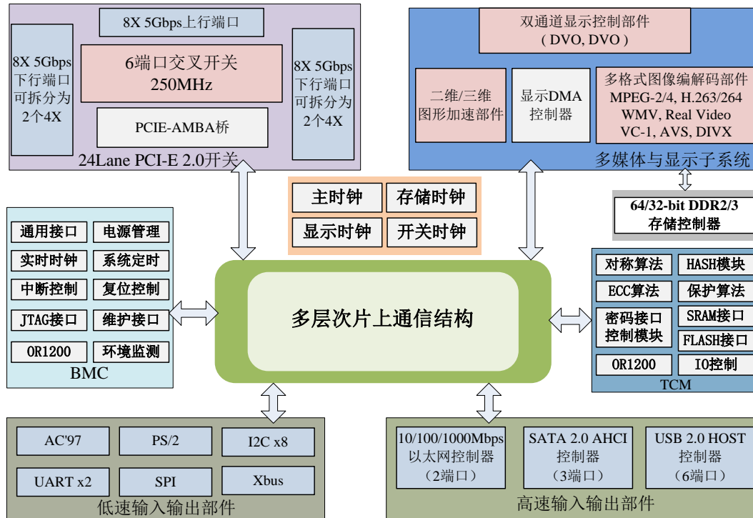
图 2 SWICH 基本结构框图
