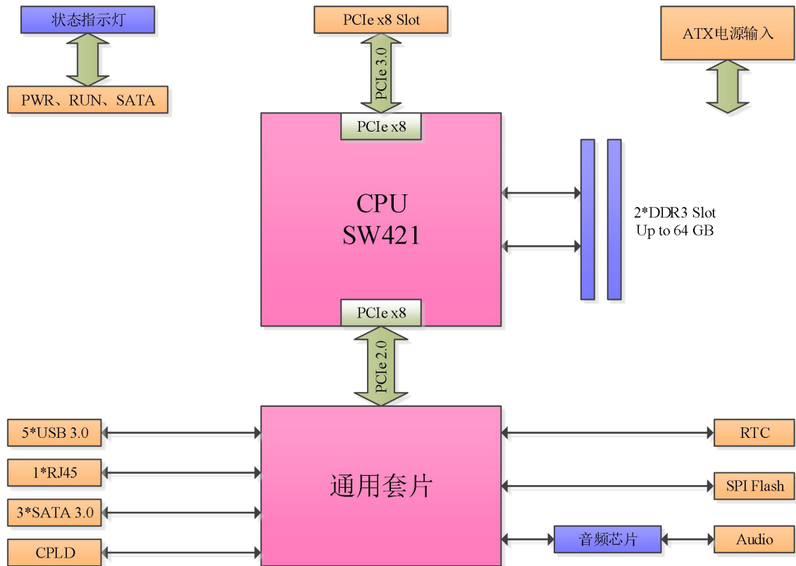
系统功能框图
